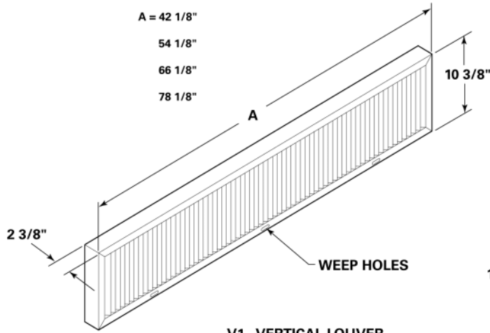
V1 - VERTICAL LOUVER
