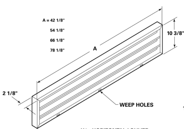
H1 - HORIZONTAL LOUVER
